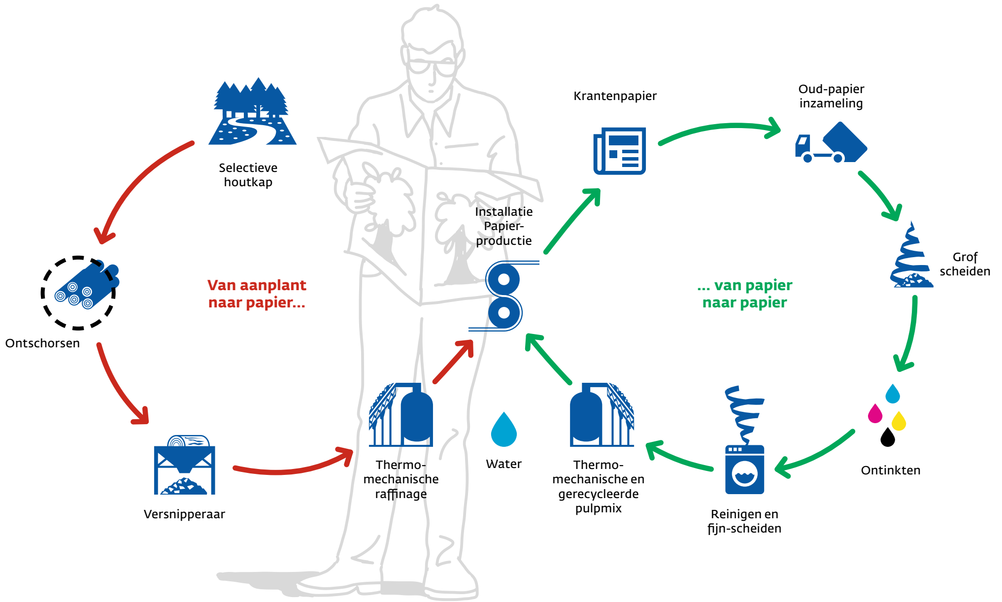
INFOGRAPHIC 11 Gesloten papierkringloop (Bron: PNEB)
