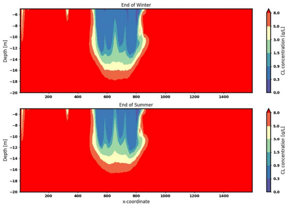
Figuur 2.47 Verticaal doorsnedeprofiel van de chloride concentratie (g Cl/l) op y=100. Boven = aan het eind van de gesimuleerde winter (eind infiltratieperiode), onder = aan het eind van de gesimuleerde zomer (eind drainage periode) voor simulatiejaar 10 van scenario 1c.
