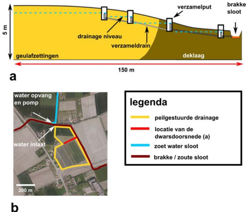
Figuur 2.5 a) Dwarsdoorsnede van het Kreekrug Infiltratie Systeem. b) Locaties peilgestuurde drainage, water inlaat/opvang en zoete en zoute sloten.
