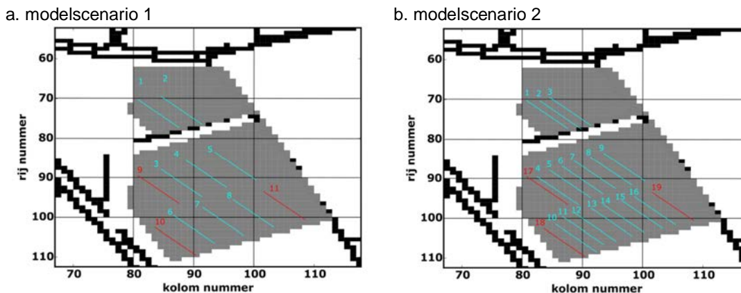
Figuur 2.33 Overzicht ligging van de drains in de verschillende modelscenario's, met a. modelscenario 1 – 11 drains, b. modelscenario 2 – 19 drains. De blauwe en rode kleur geven de draintypen aan; rode drains (type b) hebben een ander onttrekkingsdebiet dan de blauwe drains (type a).
