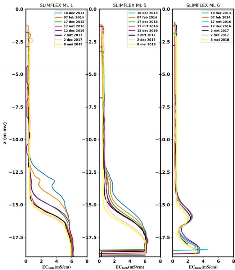
Figuur 2.16 EM-Slimflex resultaten op meetlocaties 1, 5 en 6.
