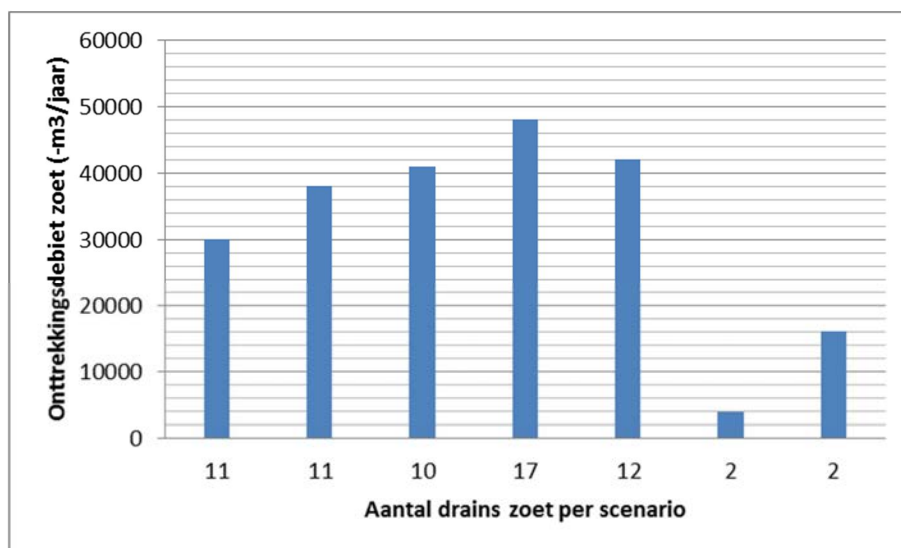
Figuur 2.40 Totale onttrekkingsdebiet zoet in m 3 /jaar uitgezet tegen het aantal draais dat zoet blijft per modelscenario.
