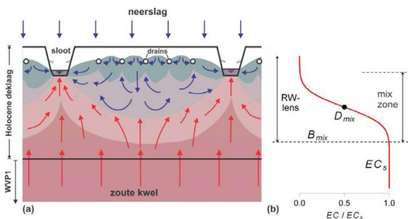
Figuur C-1: (a) Schematische weergave van een regenwaterlens zoals ze voorkomen in de zoute kwelgebieden. (b) Profiel van het zoutgehalte van het grondwater met de diepte. D_{mix} is het midden van de meng-zone waar het zoutgehalte (EC) de helft van het zoutgehalte van het kwelwater ( EC_s ) is. B_{mix} is de basis van de meng-zone waar het zoutgehalte gelijk is aan dat van het zoute kwelwater ( EC_s ). Uit De Louw et al. (2013).
