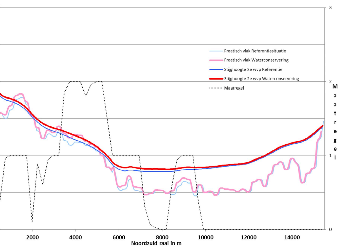
Figuur 48 Freatische stijghoogte en stijghoogten in 2 e watervoerend pakket in de referentiesituatie en bij waterconservering met stuwen.
