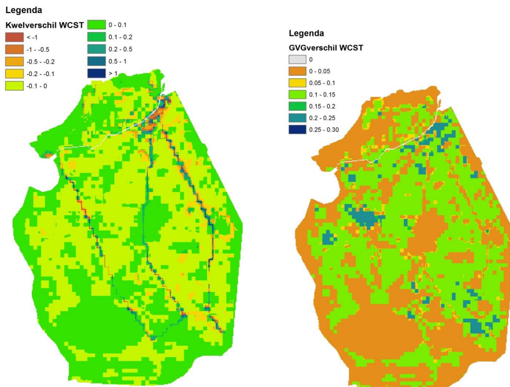
Figuur 47 Kwelderskil (links) en verschil in GVG (rechts) tussen de referentiesituatie en de situatie waarin de maatregel waterconservering met stuwen is doorgevoerd
