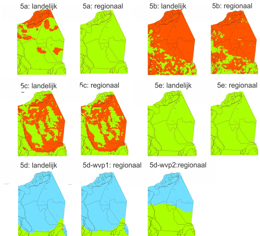
Figuur 34 Vergelijking tussen de scores van de verschillende fysische factoren voor de landelijke en regionale geschiktheidskaart: maatregel verticale ASR. Voor factor D (zoutconcentratie) is onderscheid gemaakt tussen een zout ondiep watervoerend pakket (WVP1) en een dieper zoet watervoerend pakket waar de zoetwaterbel van Hoorn zich bevindt (WVP2).
