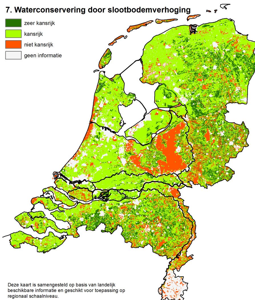
Figuur 17 Kansen voor waterconservering door slootbodemplhoging, uitgaande van de geschiktheid van de ondergrond.
