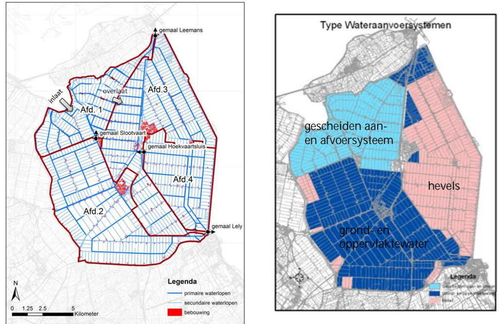
Figuur 23 a) Overzicht van de waterlopen, gemalen, inlaat en bebouwing in de Wieringermeer. b) type wateraanvoersystemen in de Wieringermeerpolder.
