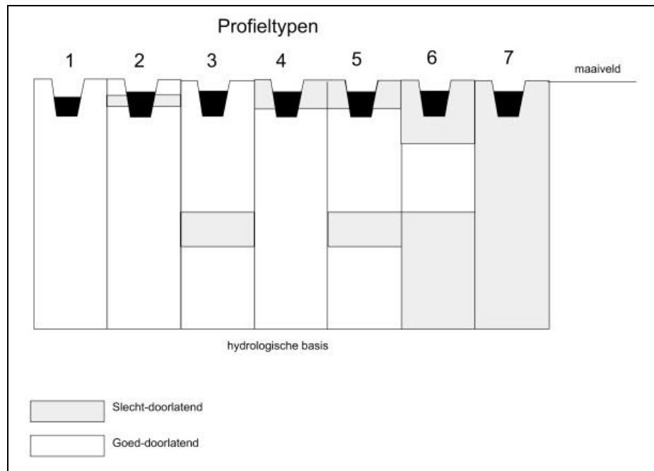
Figuur 22 Schematische indeling van leidingen ten behoeve van waterbeheer in profieltypen (bron: Massop et al., 1997)
