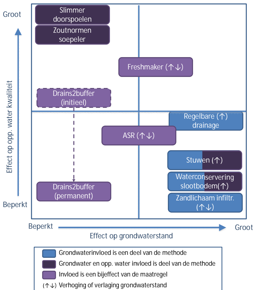
Figuur 19 Uitsplitsing van de effecten op grondwaterstand en oppervlaktewaterkwaliteit in de omgeving van de verschillende typen maatregelen.
