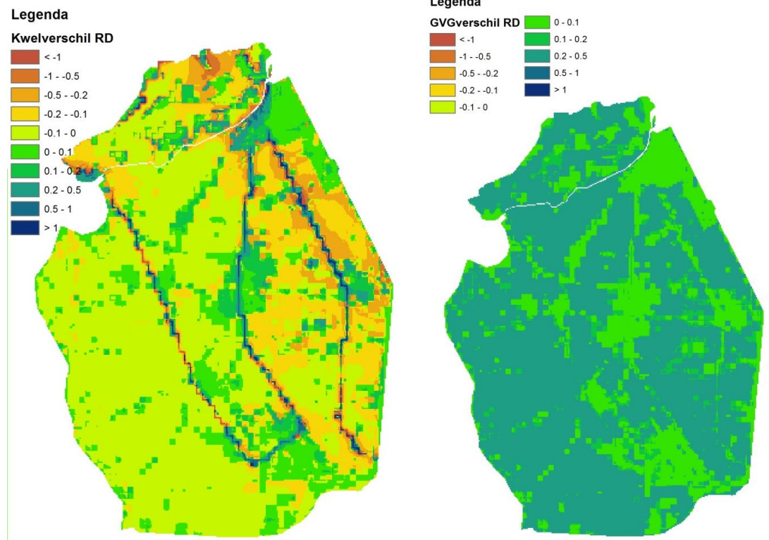
Figuur 45 Kwelverschil (links) en verschil in GVG (rechts) tussen de referentieberekening en de maatregel regelbare drainage
