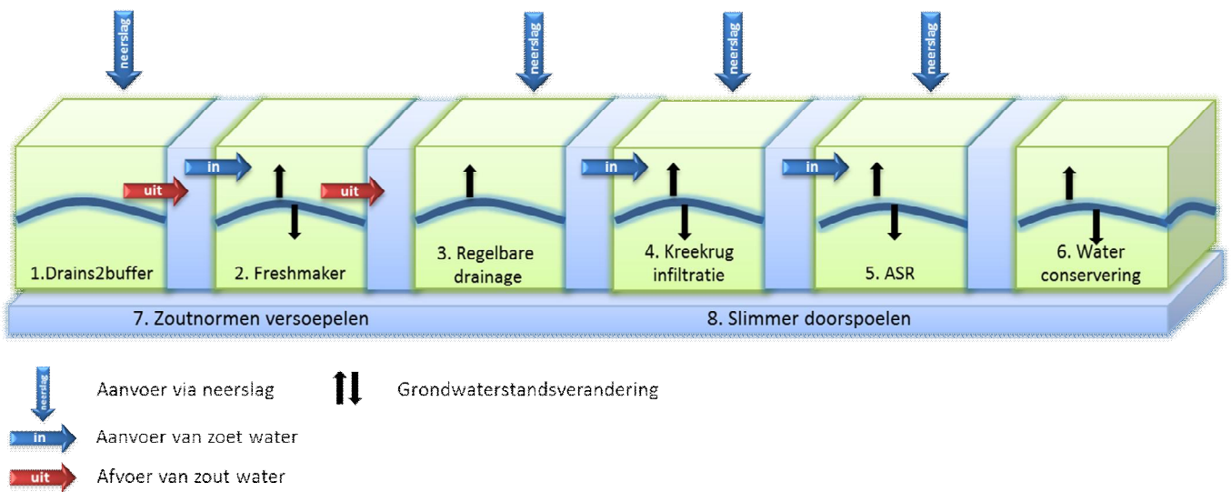
Figuur 18 Vereisten en effecten van de verschillende maatregelen in relatie tot grond- en oppervlaktewater in de omgeving.
