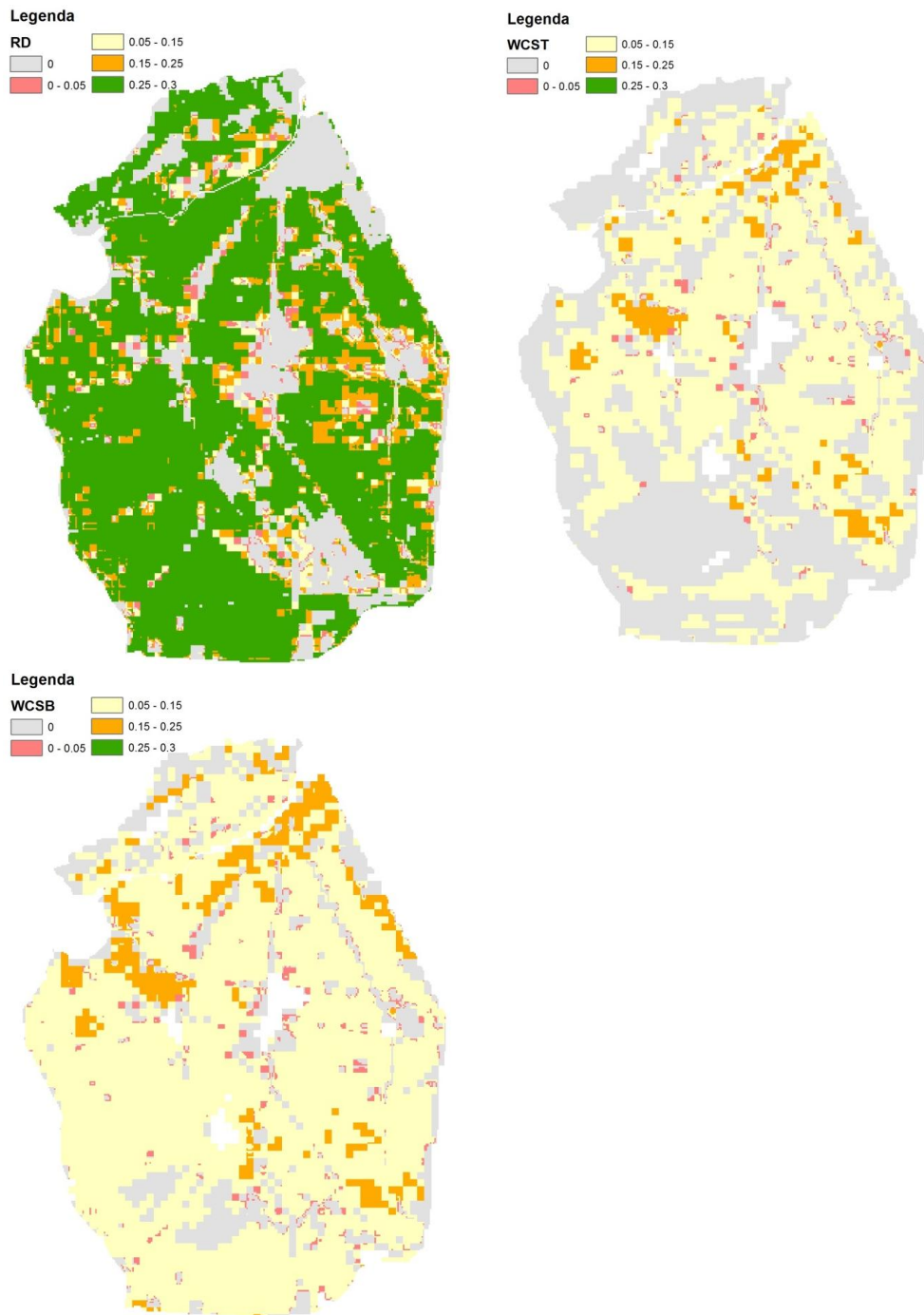
Figuur 41 GVG verhoging [m] door toepassing van Regelbare Drainage (RD, linksboven), waterconservering m.b.v. stuwen (WCST, rechtsboven) en waterconservering d.m.v. slootboderverhoging (WCSB, linksonder)
