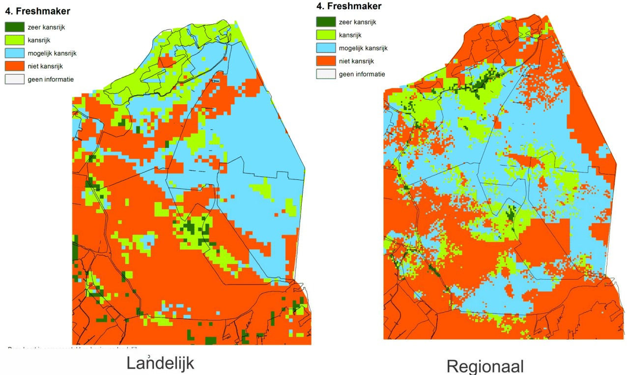
Figuur 33 Vergelijking de landelijke (links) en regionale (rechtst) geschiktheidskaart voor maatregel drains2buffer.
