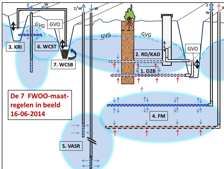
Figuur 20 Schematische visualisatie van zeven FWOO-maatregelen (Bron: De Bakelse Stroom)
