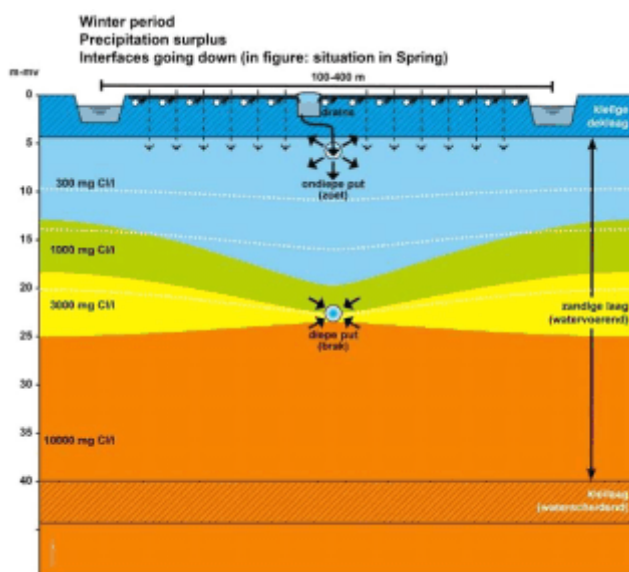
Figuur 10 Schematische weergave van de Freshmaker: toename van zoetwatervoorraad in kreekrug door injectie van zoet water en onttrekking van zout grondwater.
